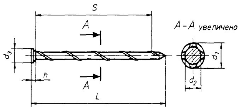
Черт. 2 Размеры, мм
